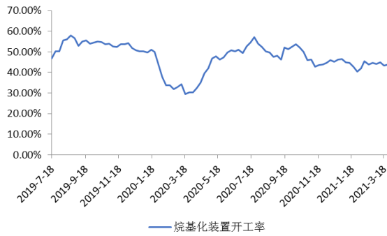
图表 10：烷基化装置开工率
