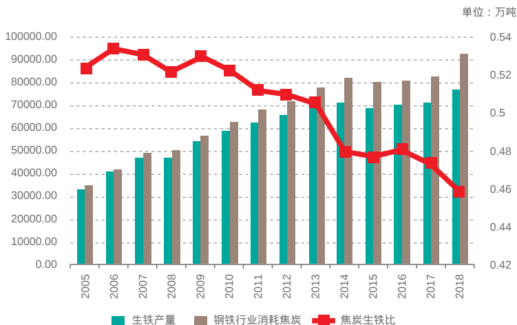
图8、2005年-2018年钢铁行业焦炭消耗量、生铁产量及比值
