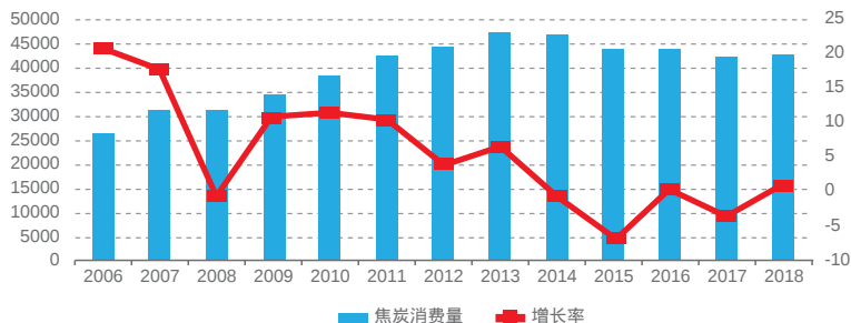
图7、2005年-2018年我国焦炭的消费量及增长率
